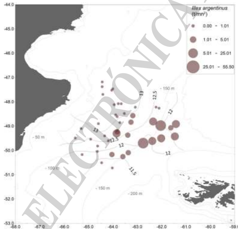
Figura 2. Illex argentinus . Campaña EH-02/24. Distribución de la abundancia relativa (t mn -2 ) por lance de pesca. Isolíneas de temperatura del agua del mar en superficie.
